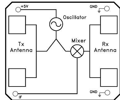
Diagram A: Block Diagram
